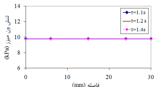
شکل (۳): نمودار تنش ون‌میزر بر روی سطح بالایی مدل بافت تنها و در ۳ زمان متفاوت در طول ۱ ثانیه دوم از زمان حل مسأله.
